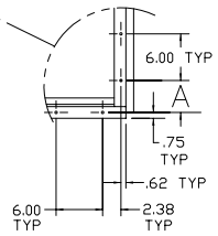
MFG DWG 096648
